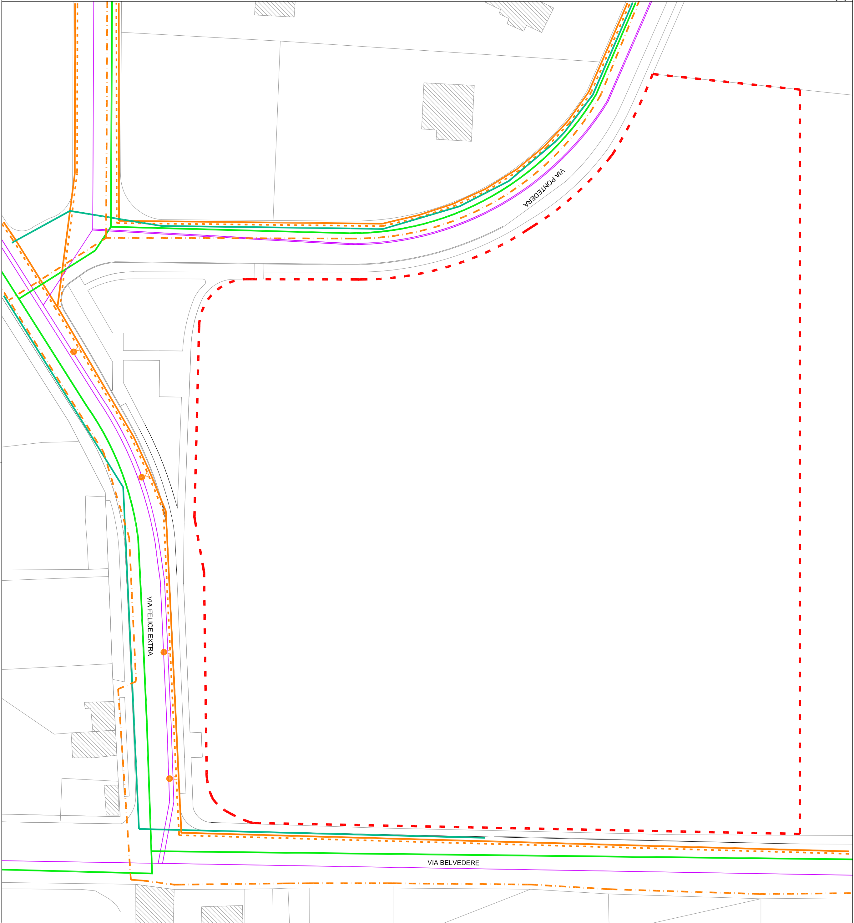
PLANIMETRIA DELLE RETI ESISTENTI - SC 1:500
